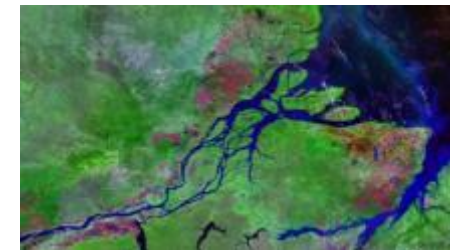
Salinity gradient
